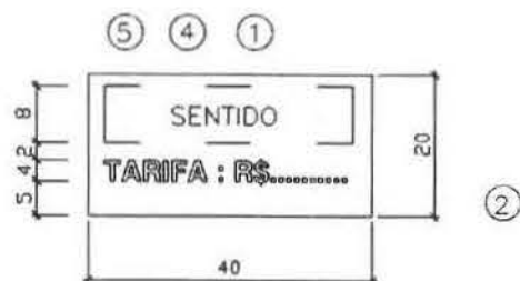
PLACA P/ O PARA-BRISA DIANTEIRO
