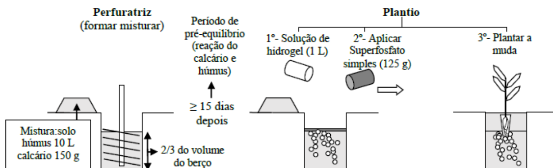
Figura 8. Ilustração esquemática do preparo do berço (calagem, adubação orgânica e inorgânica) e do plantio.
