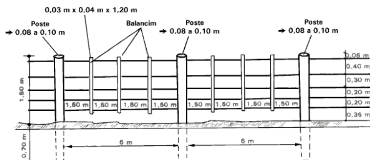
Figura 6. Croqui da cerca.
